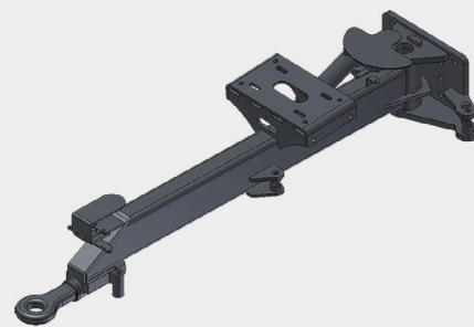
Timone sterzante idraulico automatico con occhio per gancio di traino (opzionale). Automatic hydraulic steering drawbar with towing eye (optional).
